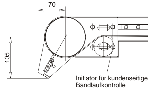
Abstreifer für TYP 362-366 Ø100
