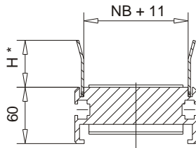
Leitbleche NB 50 und 100
