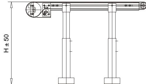
Abstützung Typ 2
