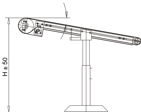
Abstützung Typ 3
