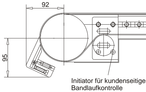
Abstreifer für TYP 360 Ø113 - Ø123
