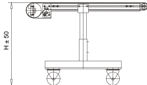
Abstützung Typ 4
