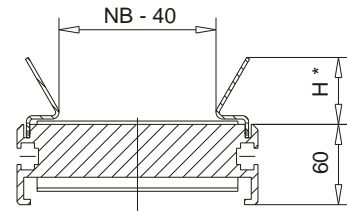
Leitbleche ab NB 150
