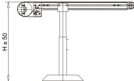
Abstützung Typ 1
